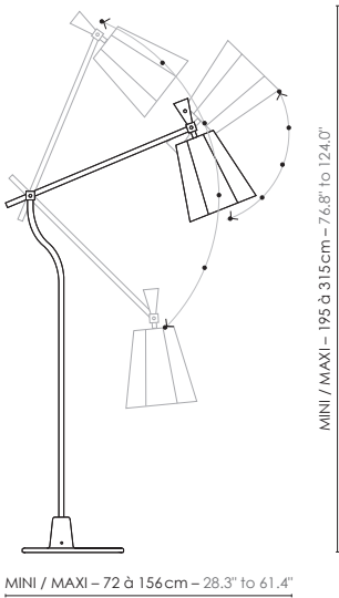
6 positions de bras et 5 d’abat-jour 6 arm positions and 5 lampshade positions
