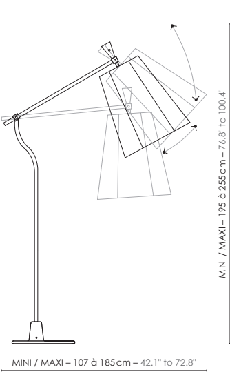
2 positions de bras et d’abat-jour 2 arm and lampshade positions
